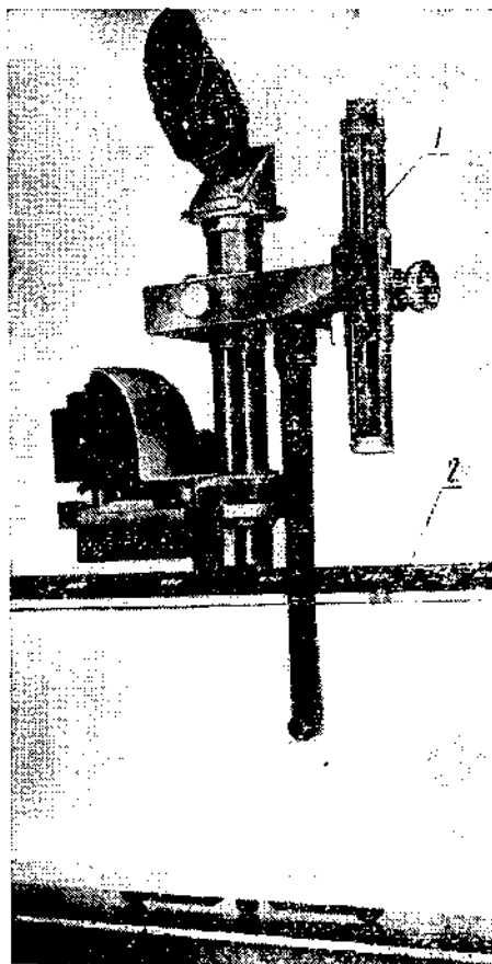
Линейка снабжена графическим устройством 1 (рис. 2), присоединяемым к измерительной каретке. Перемещая каретку по проверяемой поверхности, воспроизводят графически ее профиль наколами иглы на миллиметровой бумаге 2, которая прикреплена к доске, привинчиваемой к корпусу прибора.
