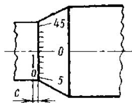
Рис. 3. Определение расстояния s от края торца конической части барабана до нулевого штриха шкалы стебля
